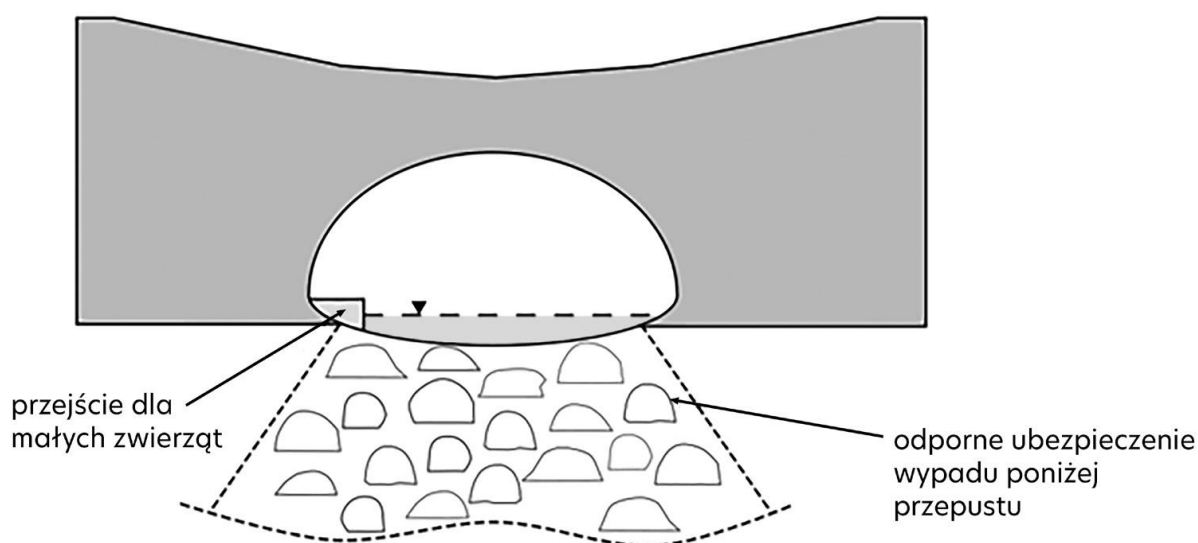
Rys. 110. Schemat przepustu z przelewem górnym
