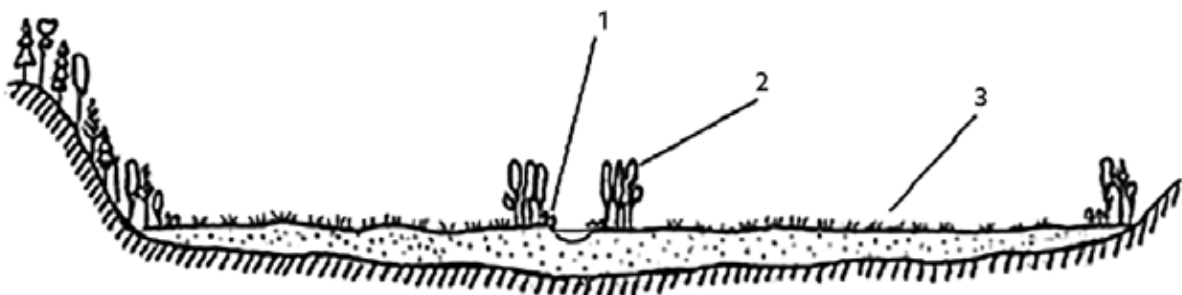
Rys. 10. Zabudowa biologiczna dolnej części cieku przy korelacji na średnią wielką wodę: 1 – pasy korytowe, 2 – pasy przykorytowe, 3 – trwałe użytki zielone [Prochal 1968].
