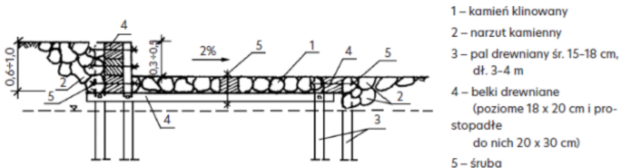
Rys. 46. Próg drewniano-kamienny [Wołoszyn 1994].
