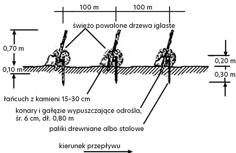
Rys. 59. Schemat żywych ostróg pośrednich [Begemann i Schiechtl 1999].
