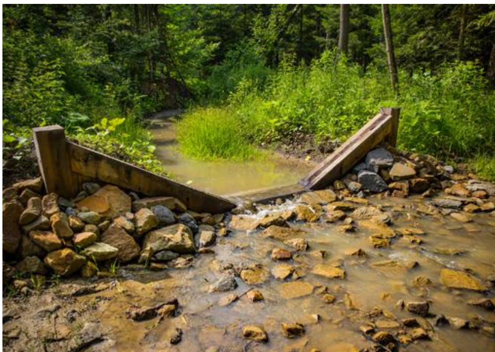
Fot. 38. Piętrzenie stałe – ścianka szczelna podparta bystrzem w Nadleśnictwie Maskulińskie, 2015 (archiwum CKPŚ).
