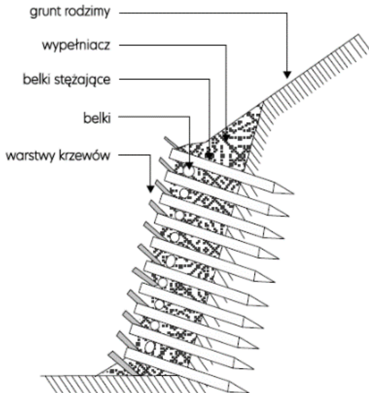
Rys. 81. Przekrój poprzeczny kaszycy [Begemann i Schiechl 1999].
