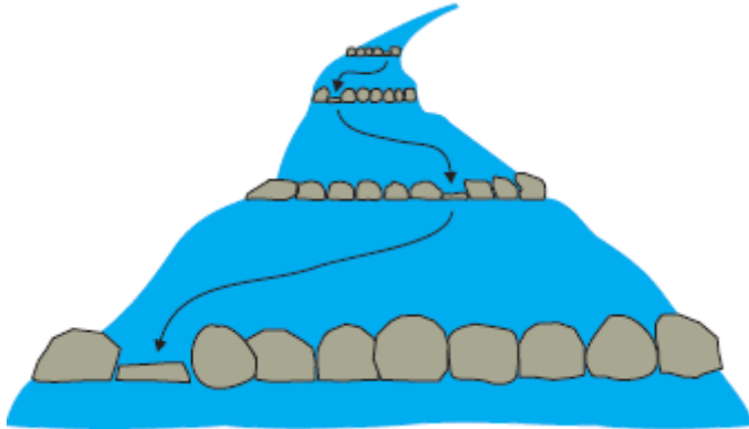
Rys. 107. Progi kamienne z naprzemiennymi przelewami
