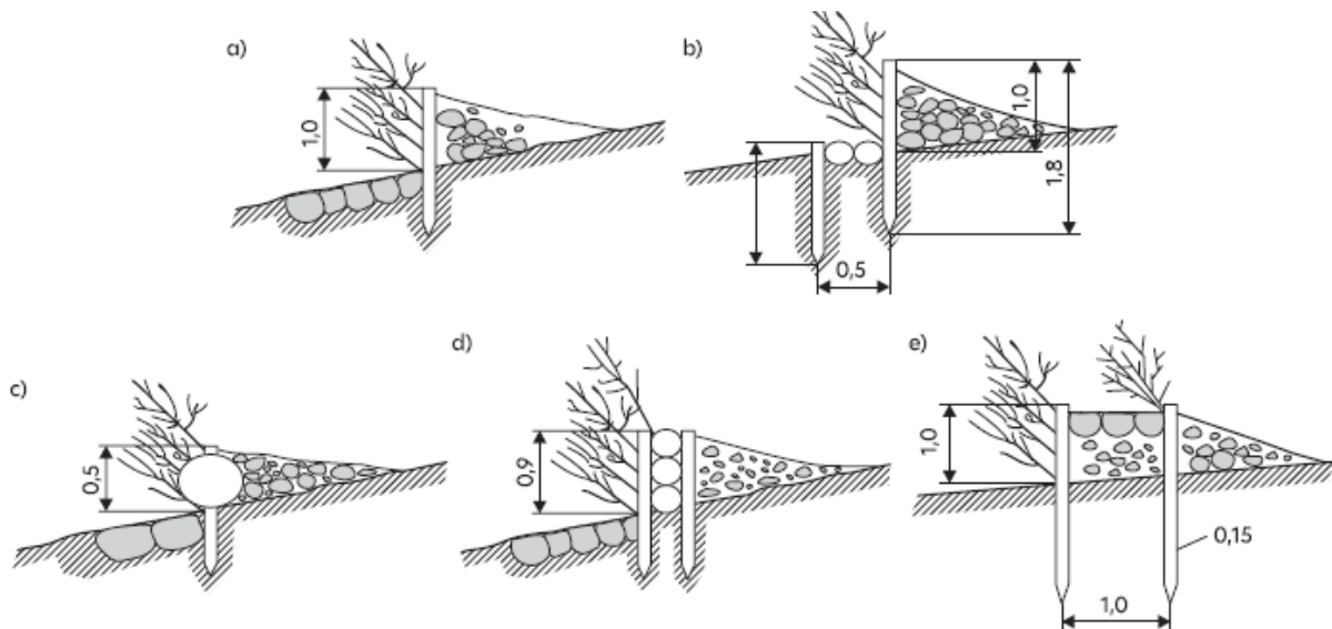
Rys. 99. Płotki drewniano-ziemne z nasadzeniami: a, d, c, d – pojedyncze, e – podwójne [opracowano na podstawie: Prochal 1968]
