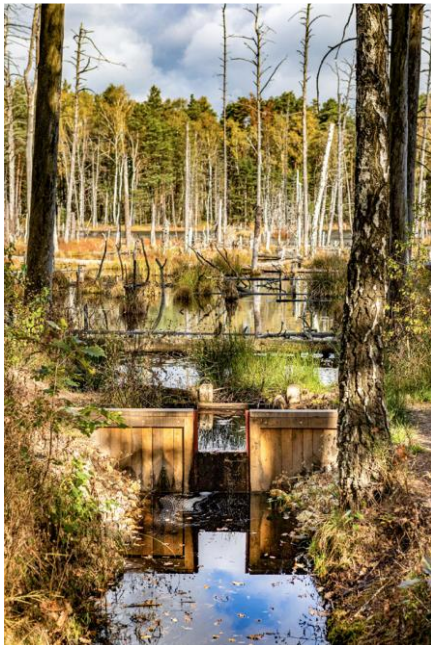
Fot. 34. Zastawki drewniane w Nadleśnictwie Celestynów (fot. J. Smarczewski, 2021).
