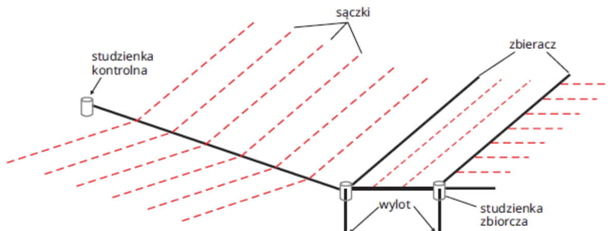
Rys. 49. Przykładowy schemat sieci drenarskiej (rys. L. Książek).
