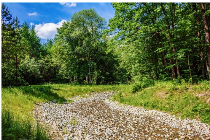
Fot. 90. Bystrze o zwiększonej szorstkości w miejscu rozebranego betonowego jazu w Nadleśnictwie Krasiczyn, przywracające ciągłość biologiczną cieku (archiwum CKPŚ).
