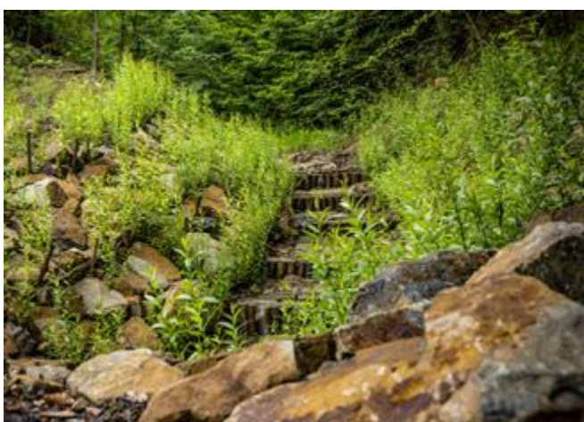
Fot. 77. Zabezpieczony faszyną narzut kamienny z nasadzeniami wierzbowymi, Nadleśnictwo Baligród (archiwum CKPŚ).
