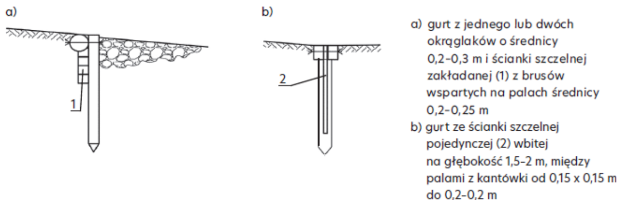
Rys. 48. Gurty [Biedroń 2018, na podstawie: Wołoszyn i in. 1994].
