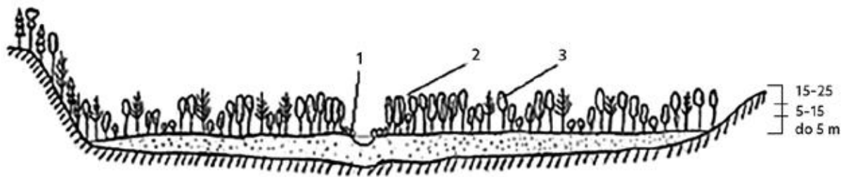
Rys. 10. Zabudowa biologiczna dolnej części cieku przy korelacji na średnią wielką wodę: 1 – pasy korytowe, 2 – pasy przykorytowe, 3 – trwałe użytki zielone [Prochal 1968].
