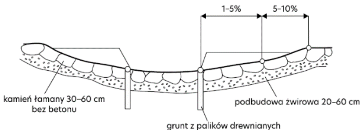
Rys. 85. Szkic brodu z Nadleśnictwa Łosie.
