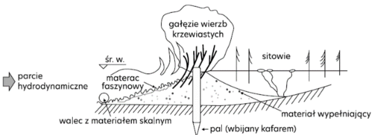
Rys. 84. Tama faszynowa [Begemann i Schiechl 1999].
