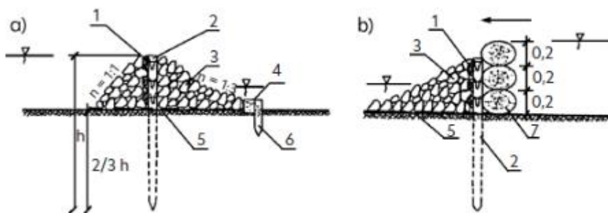
Rys. 42. Progi o konstrukcji mieszanej [Jędryka 2006].
