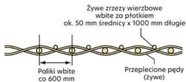
Rys. 75. Schemat płotka plecionego [Krukowski 2006].
