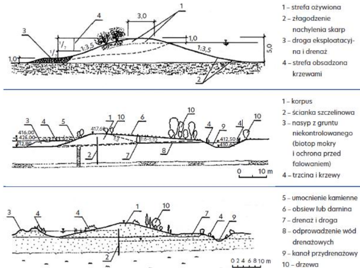
Rys. 18. Niskie zapory ziemne i wały przeciwpowodziowe dostosowane do wymagań ekologicznych [Żbikowski i Żelazo 1993].
