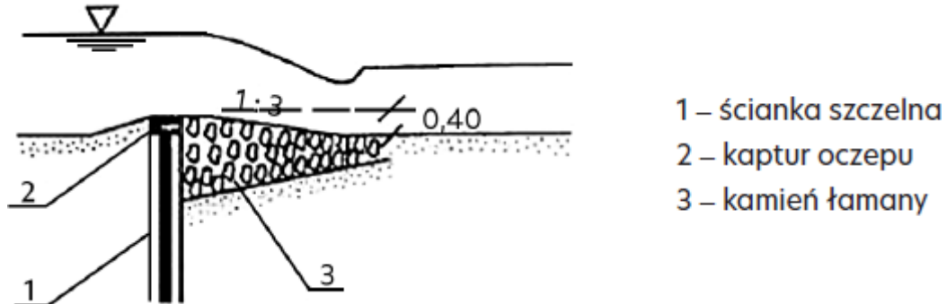
Rys. 36. Próg ze ścianki szczelnej [Dębski 1971].
