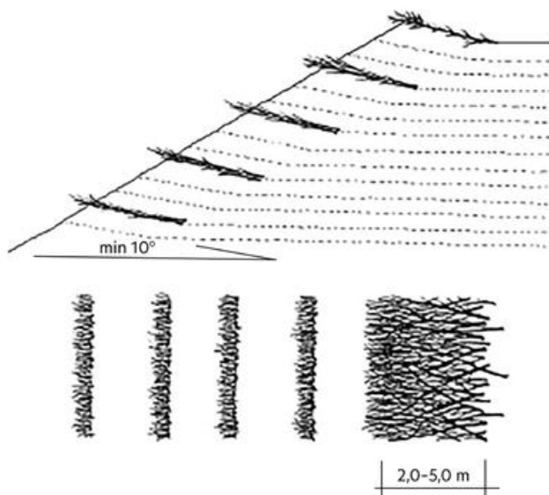
Fot. 64. Krzewiaste umocnienia tarasowe na skarpie/osuwisku [Begemann i Schiechtl 1999].
